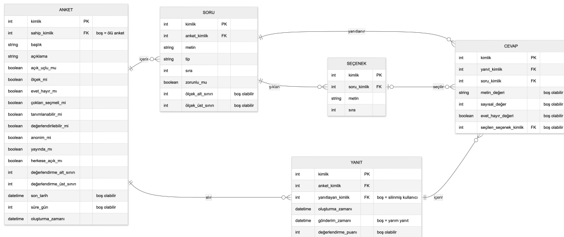
ŞEKİL 1: ANKET İÇERİĞİ VE YANIT MODELİ
