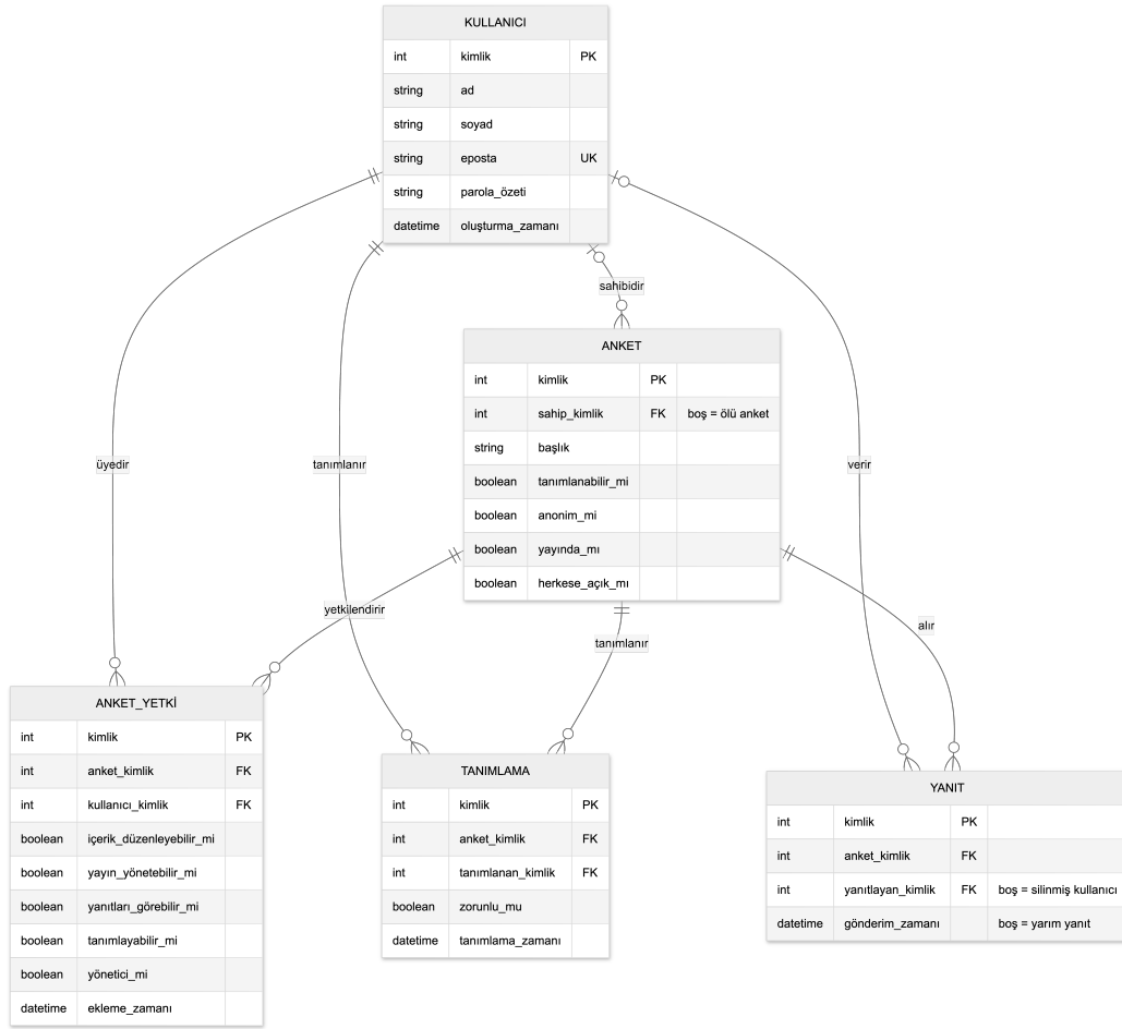
ŞEKİL 2: KULLANICI VE ERİŞİM MODELİ
